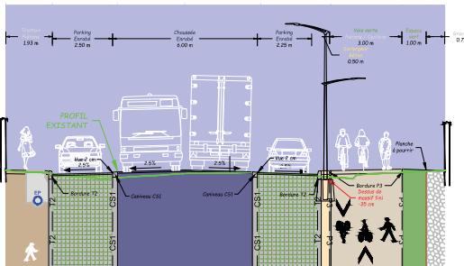
Profil entravers type - CC Ech : 1/100
