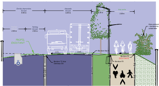
Profil entravers type - CC Ech : 1/100
