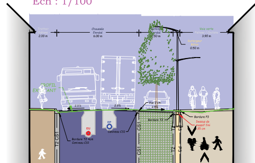
Profil entravers type - EE Ech : 1/100
