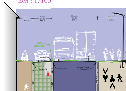
Profil entravers type - EE Ech : 1/100
